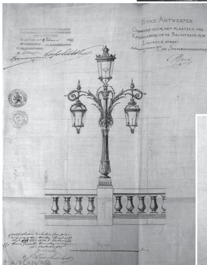
Afbeelding 3-4: Ontwerpen voor publieke verlichting in de Antwerpse Kruidtuin (1877) en een combinatie van lantaarn en urinoir te plaatsen op de Grote Markt (1878). (Stadsarchief Antwerpen)
